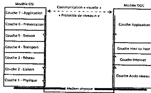
Figure 26.2 Les modèles OSI et DOD
