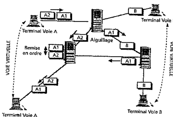
Figure 22.5 Commutation de paquets et circuits virtuels
