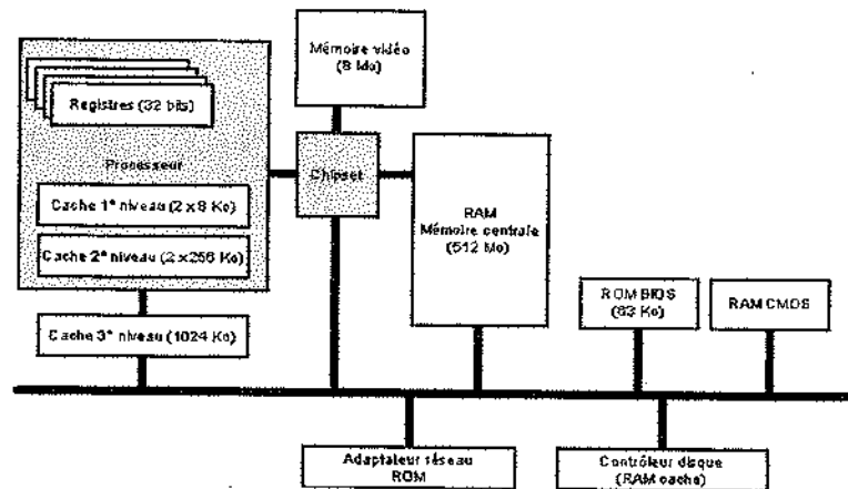
Figure 11.3 Usage des mémoires électroniques (valeurs indicatives)
