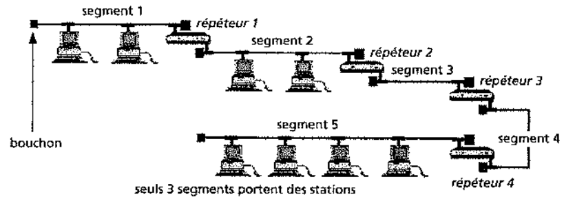
Figure 25.10 Ethernet et la règle des 5-4-3
