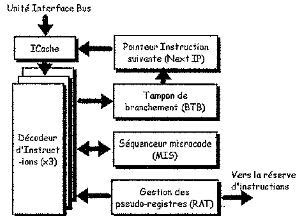
Figure 10.7 L'unité de recherche-décodage
