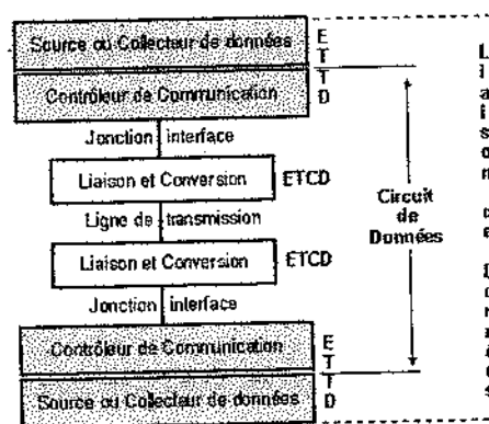
Figure 21.14 Composants de la liaison téléinformatique
