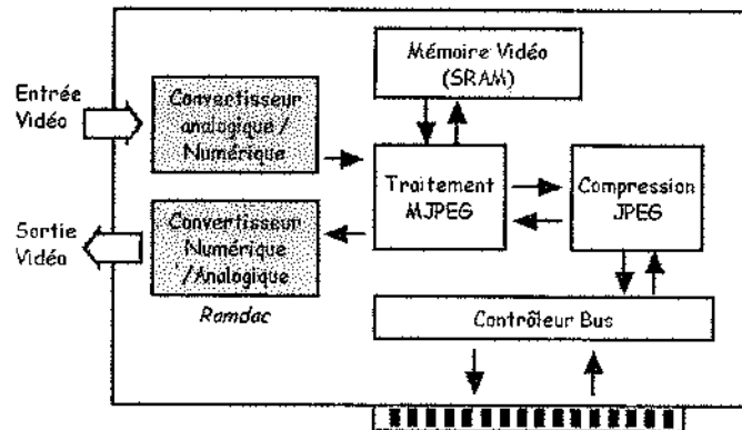
Figure 19.4 Carte Vidéo
