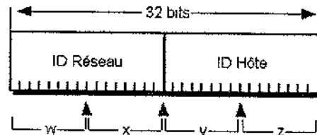
Figure 24.2 Informations contenues dans l'adresse IP (Exemple en classe B)
