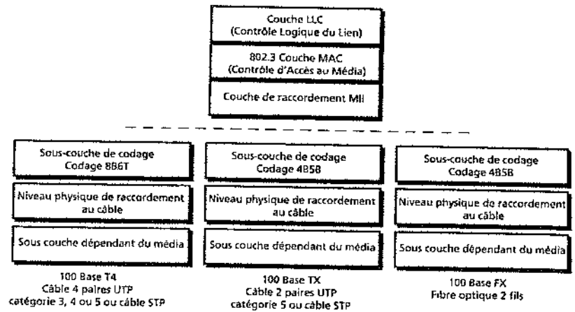
Figure 25.15 Décomposition de la norme Fast Ethernet
