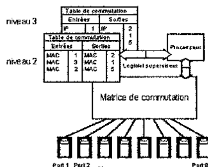
Figure 26.9 Le commutateur
