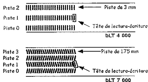
Figure 12.9 Les formats DLT 4000 et 8000
