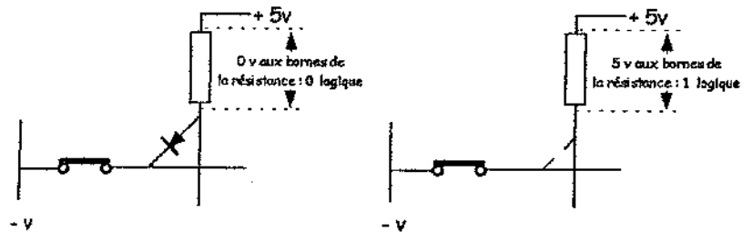
Figure 11.17 Principe de fonctionnement de la PROM
