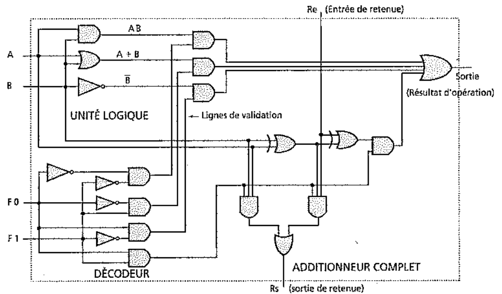
Figure 7.6 Exemple simple d'UAL 1 bit
