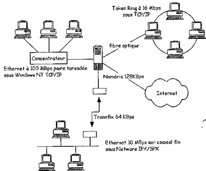
Figure 26.1 Exemple d'interconnexion de réseaux
