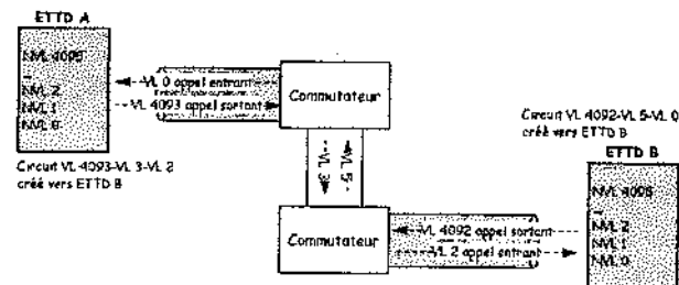
Figure 23.8 Établissement d'un circuit virtuel
