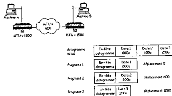
Figure 24.16 Le MTU et la fragmentation
