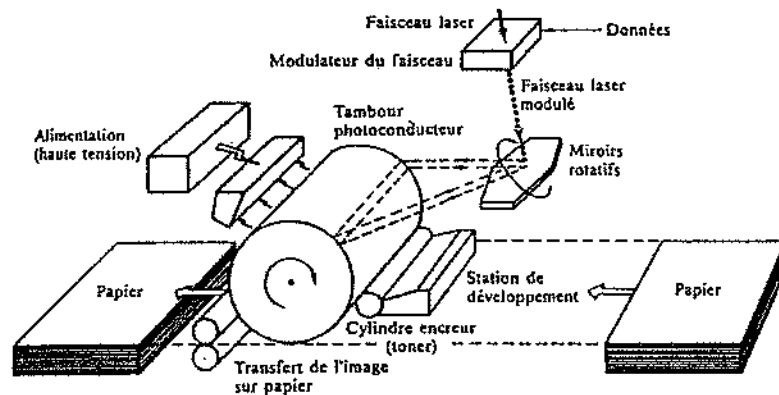
Figure 18.7 Principe de l'imprimante laser
