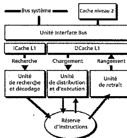
Figure 10.6 La réserve d'instructions
