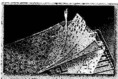
Figure 20.7 Matrice de clavier à contacts sérigraphiés
