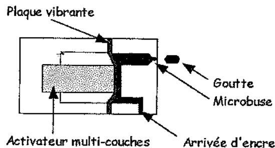
Figure 18.4 Principe de la goutte à la demande
