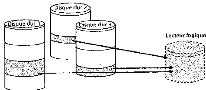
Figure 16.4 Agrégat de partitions
