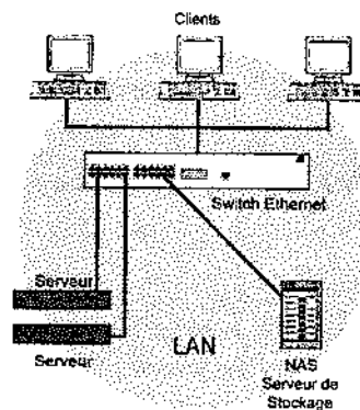
Figure 27.2 Stockage en réseau – serveur NAS
