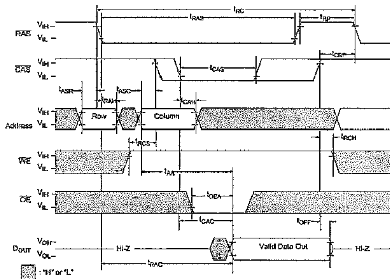
Figure 11.12 Chronogramme d'accès en mémoire
