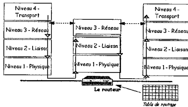
Figure 26.10 Rôle du routeur
