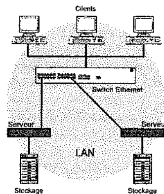
Figure 27.1 Stockage à attachement direct DAS
