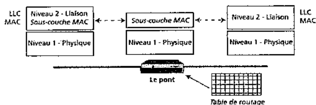
Figure 26.6 Rôle du pont
