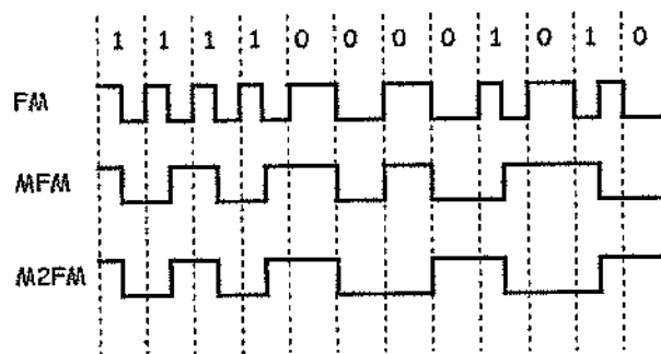
Figure 13.6 Modes d'enregistrements
