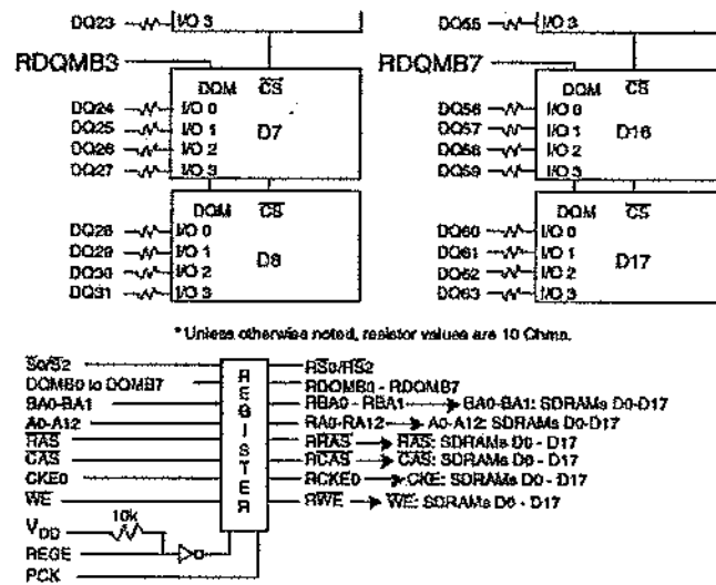
Figure 11.11 Extrait d'une implantation SDRAM 133 (doc. IBM)
