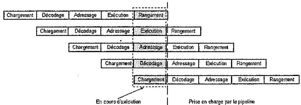
Figure 10.3 Fonctionnement du pipeline
