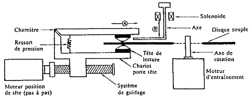
Figure 15.4 Lecteur de disquette
