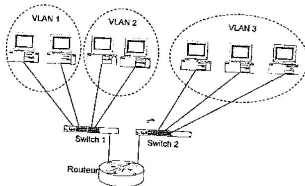
Figure 26.16 Réseaux VLAN
