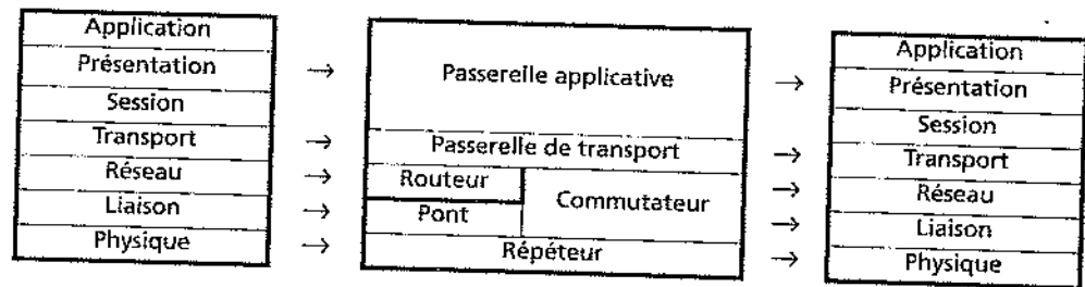
Figure 26.3 Les différentes passerelles
