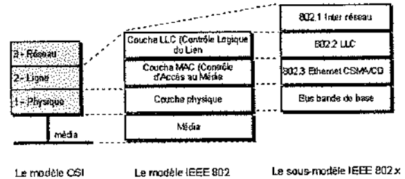
Figure 25.4 Normalisation des trames Ethernet
