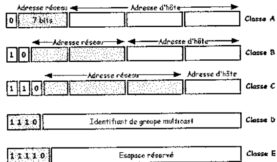
Figure 24.3 Les classes d'adresses IP
