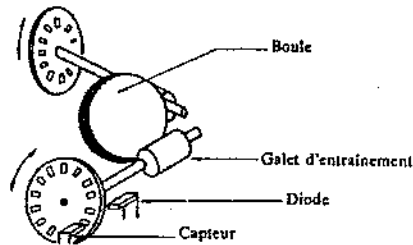
Figure 20.12 Principe de la souris opto-mécanique
