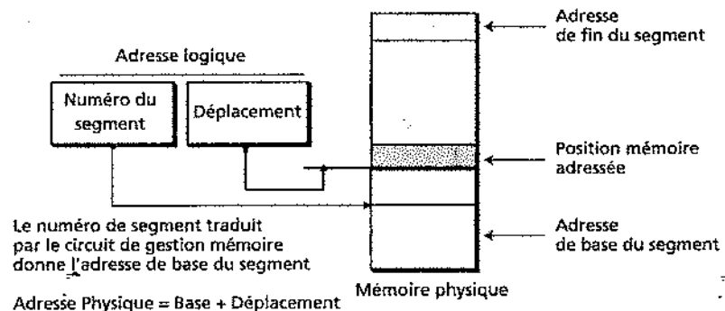
Figure 17.5 Principe de l'adressage d'une position mémoire
