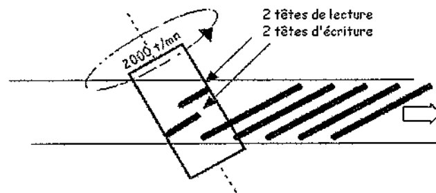
Figure 12.7 Enregistrement hélicoïdal
