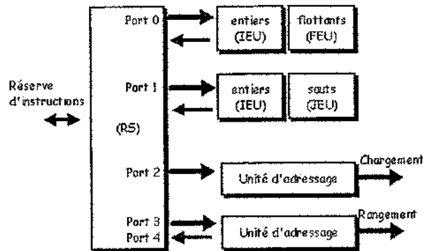
Figure 10.8 L'unité de répartition
