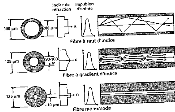
Figure 22.16 Types de fibres optiques
