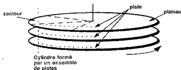
Figure 13.4 Plateaux, secteurs et pistes
