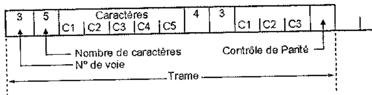
Figure 21.13 Multiplexage temporel statistique
