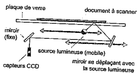
Figure 20.15 Principe du scanner à plat
