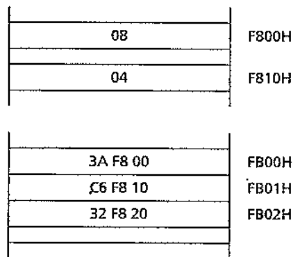
Figure 7.9 État de la mémoire avant exécution du programme
