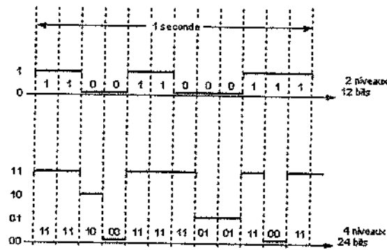
Figure 21.2 Valence et débit binaire
