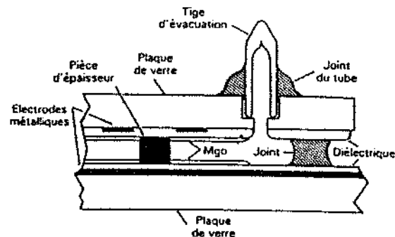
Figure 19.7 Principe de l'écran plasma
