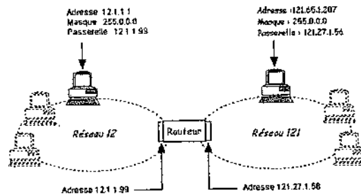
Figure 24.15 Rôle du routeur
