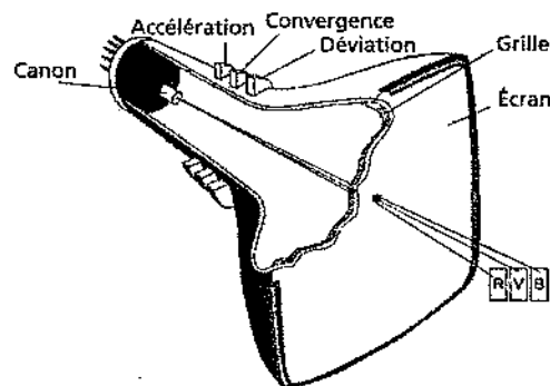
Figure 19.1 Coupe d'un TRC
