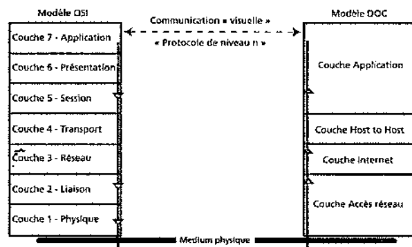
Figure 24.1 Les modèles OSI et DOD
