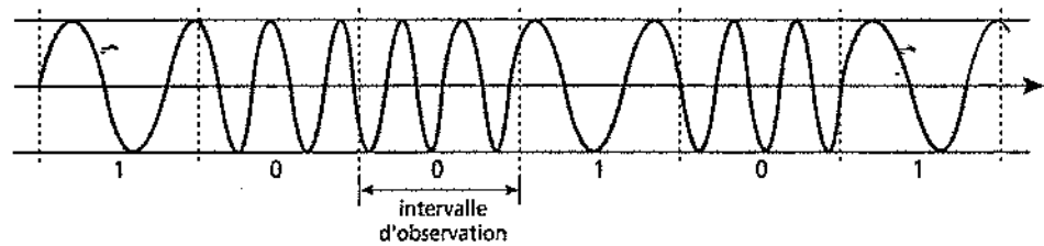
Figure 21.4 La modulation de fréquence (autre méthode)
