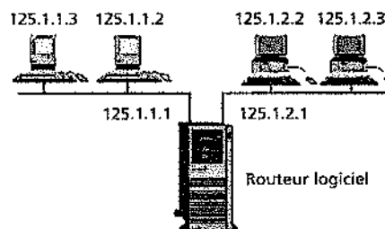
Figure 24.5 Routage par subnetting de réseaux IP
