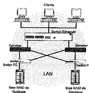
Figure 27.5 Réseau de stockage – SAN
