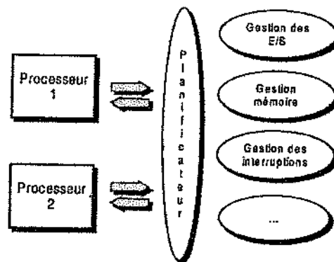
Figure 10.14 Le traitement symétrique
