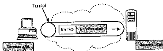
Figure 26.18 Génération de l'en-tête - tunneling
