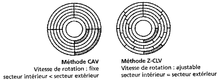
Figure 14.12 Méthodes CAV et Z-CLV
