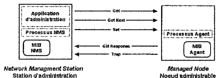
Figure 26.27 Messages échangés entre Manager et Agent
