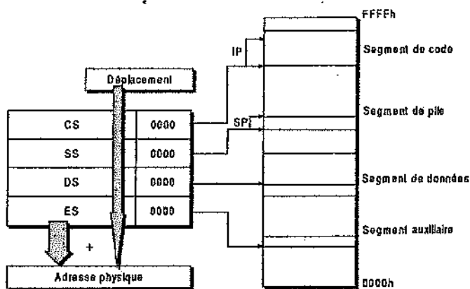
Figure 8.1 Adressage du 8086
