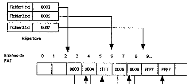
Figure 16.9 Exemple de FAT
