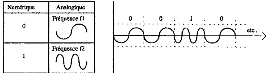
Figure 21.3 La modulation de fréquence
