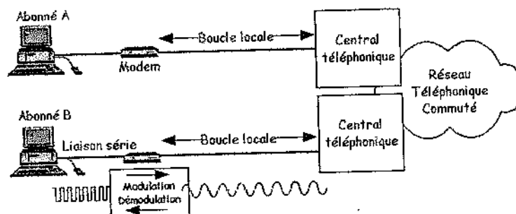
Figure 22.20 Rôle et place du MODEM
