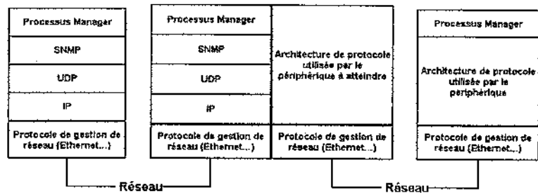
Figure 26.25 Rôle du Proxy Agent
