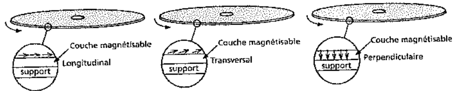
Figure 13.1 Technologies d'enregistrement
