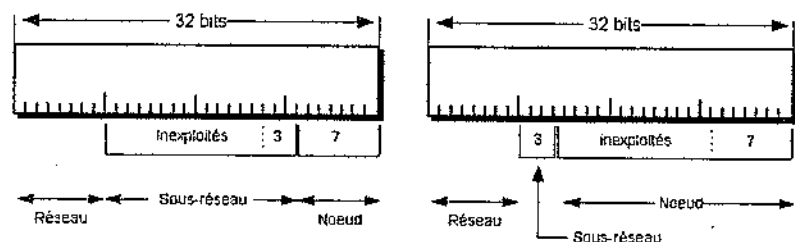
Figure 24.7 Réseaux - Sous-réseaux
