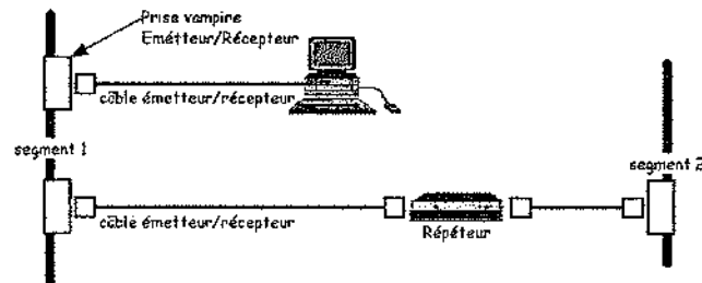
Figure 25.11 Ethernet épais 10 Base-5
