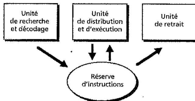
Figure 10.5 Les trois moteurs du Pentium Pro
