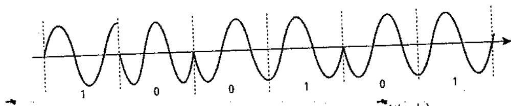
Figure 21.7 La modulation de phase (autre méthode)
