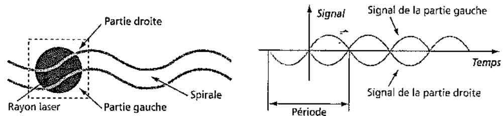
Figure 14.11 Asservissement des pistes sur un CD
