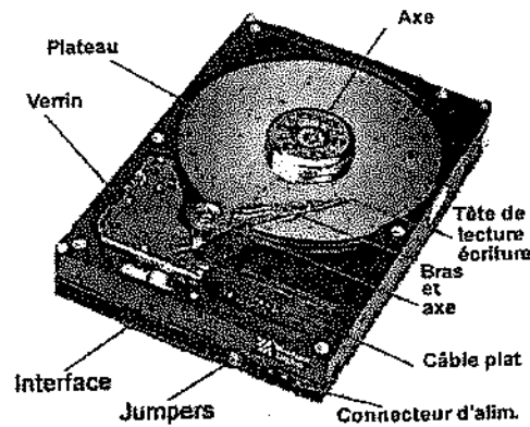
Figure 13.2 Éclate d'un disque dur
