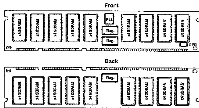
Figure 11.10 Implantation de puces de SDRAM 133 sur une barrette (doc. IBM)
