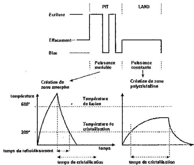
Figure 14.6 Écriture en transition de phase
