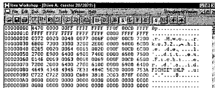
Figure 16.20 Secteur 0 – Master Boot Record du disque dur
