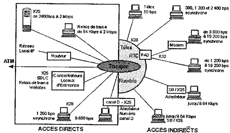
Figure 28.6 Accès Transpac
