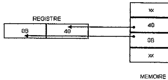
Figure 16.8 Format Intel de chargement des registres
