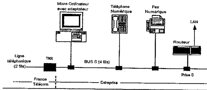
Figure 28.3 Terminaux Numéris
