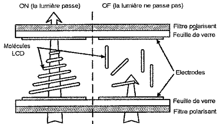
Figure 19.5 Principe de l'écran à cristaux liquides
