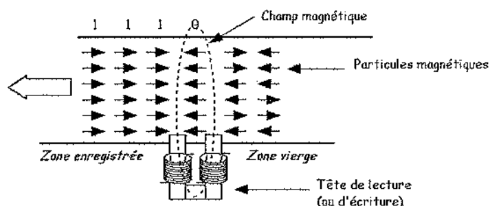
Figure 12.1 Structure de la bande magnétique
