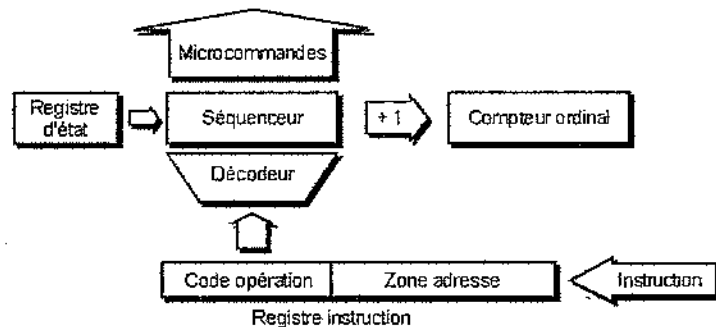
Figure 7.5 Schéma simplifié de l'unité de commandes
