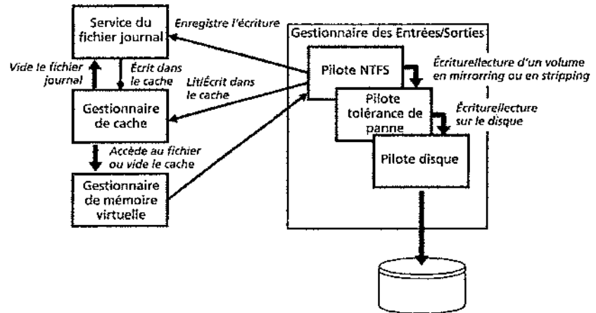
Figure 16.22 Les composants NTFS et exécutifs de Windows NT
