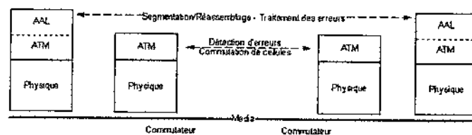
Figure 23.15 Rôle des couches ATM
