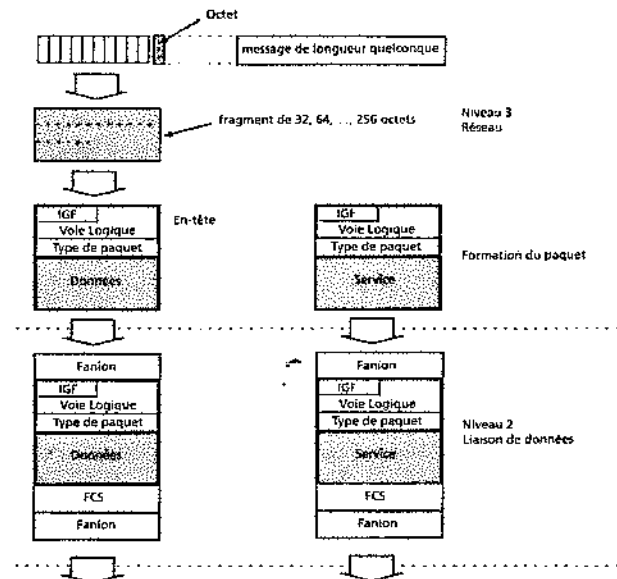
Figure 23.12 La formation des paquets sous Transpac
