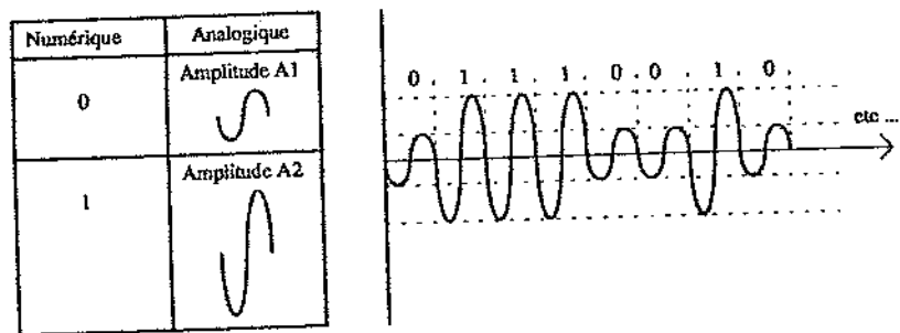
Figure 21.5 La modulation d'amplitude
