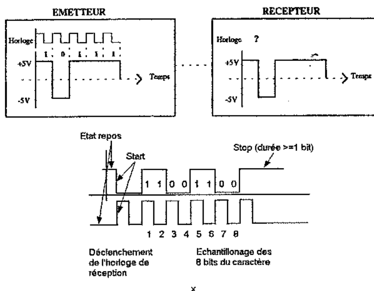
Figure 21.10 Le problème de la synchronisation
