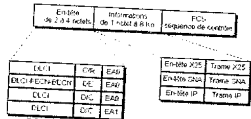
Figure 23.14 Format des paquets en relais de trame
