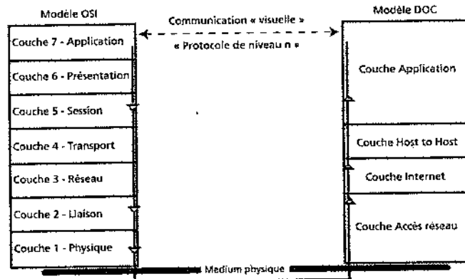
Figure 22.27 Les modèles OSI et DOD.
