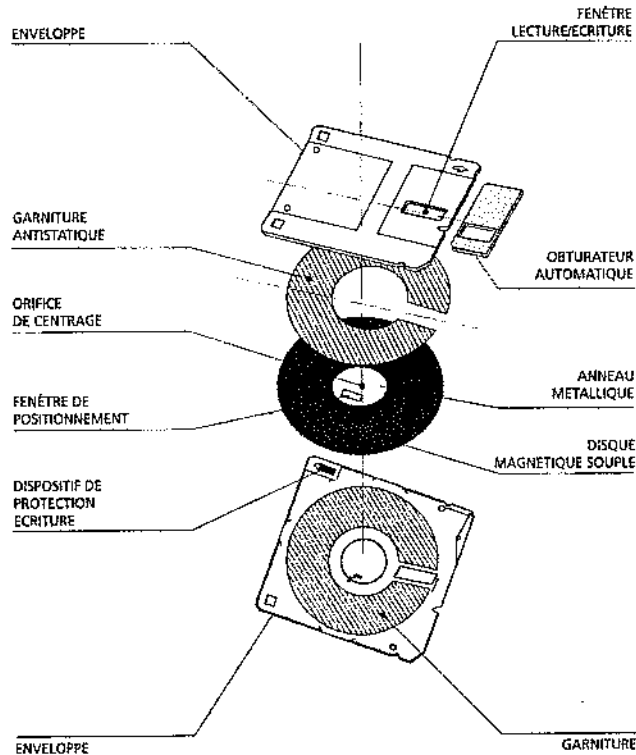
Figure 15.2 Coupe d'une disquette 3" 1/2
