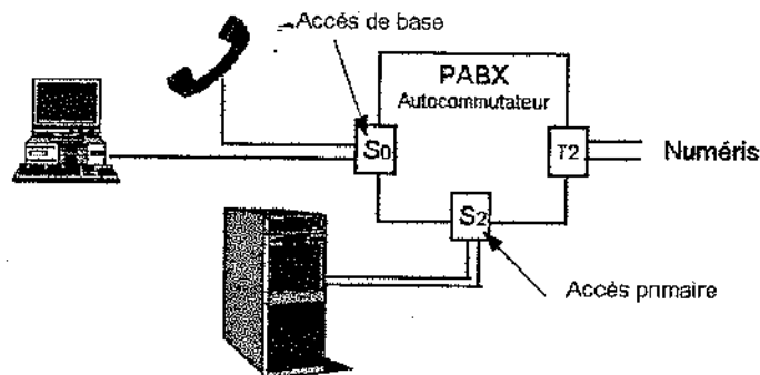
Figure 28.4 Accès Numéris
