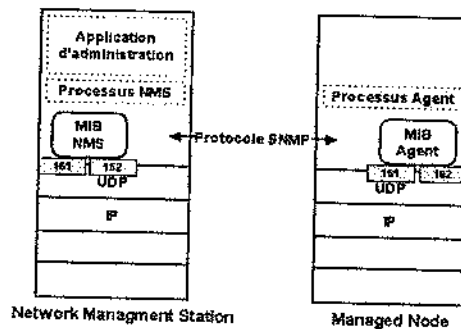
Figure 26.24 Constituants de SNMP
