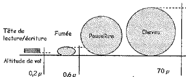
Figure 13.5 Tailles des impuretés et hauteur de vol des têtes
