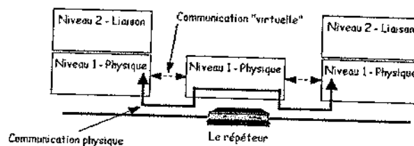
Figure 26.4 Rôle du répéteur
